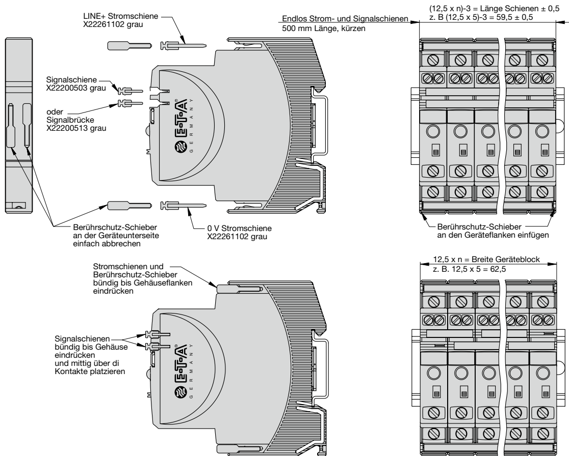
Darstellung 5 ESX10-TB mit Stromschiene und Signalbrücke
