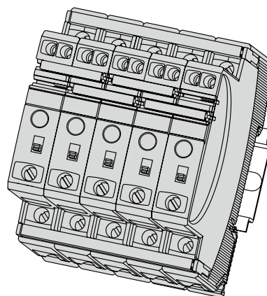
Darstellung 5 ESX10-TB mit Stromschiene und Signalbrücke
